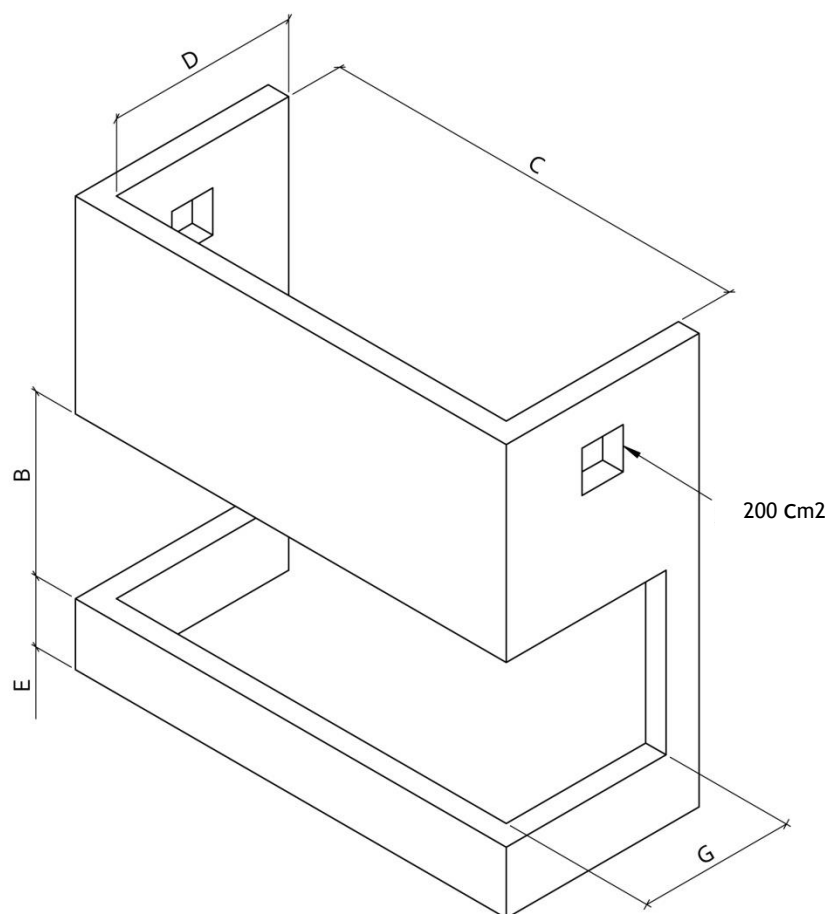
Størrelser for innbygging av Superior 1100 B
